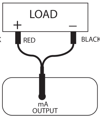
Fig. 2 mA Source Output
